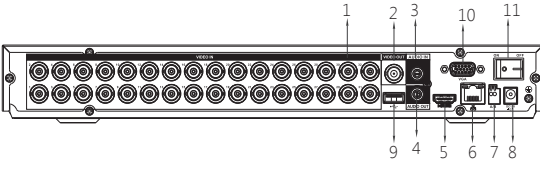
DH-XVR4232AN-X
