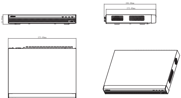
DH-XVR4232AN-X
